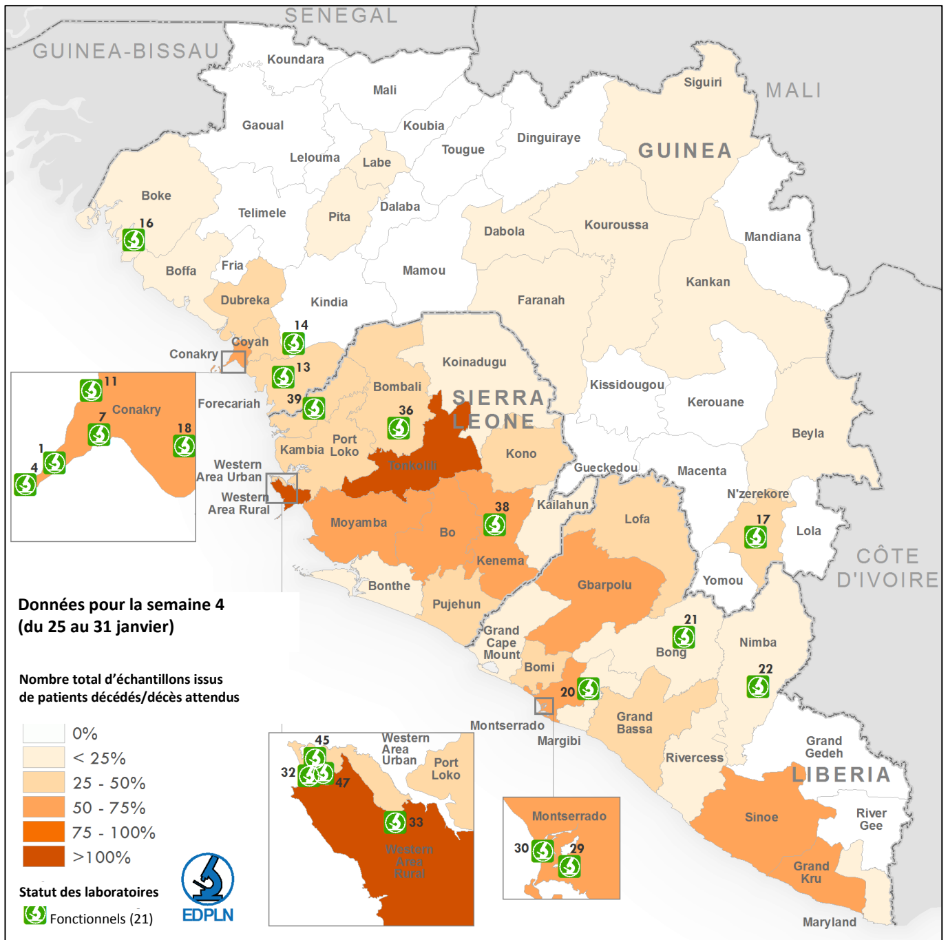
Figure 4 : Emplacement des laboratoires et répartition géographique des échantillons provenant de patients décédés en Guinée, au Libéria et en Sierra Leone la semaine précédant le 31 janvier 2016
